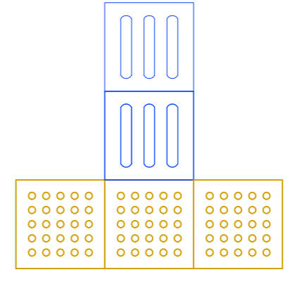
05 PISO TÁTIL - ALERTA FINAL SEM ESCALA
