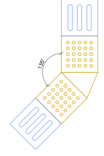
06 PISO TÁTIL - 135° SEM ESCALA
