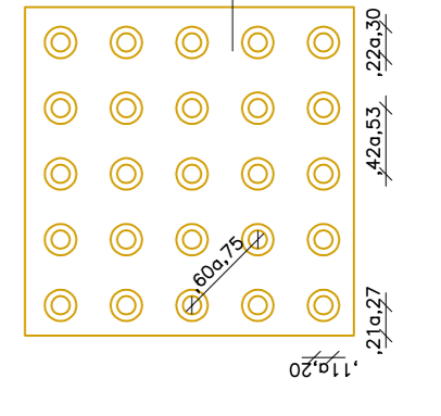
03 PISO TÁTIL DIRECIONAL SEM ESCALA
